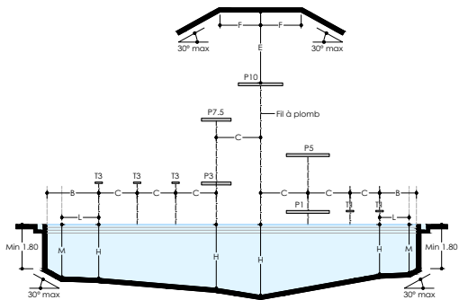
COUPE TRANSVERSALE
